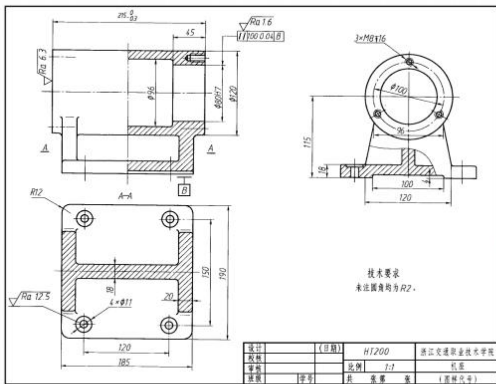
图 5-78 机座的零件图
