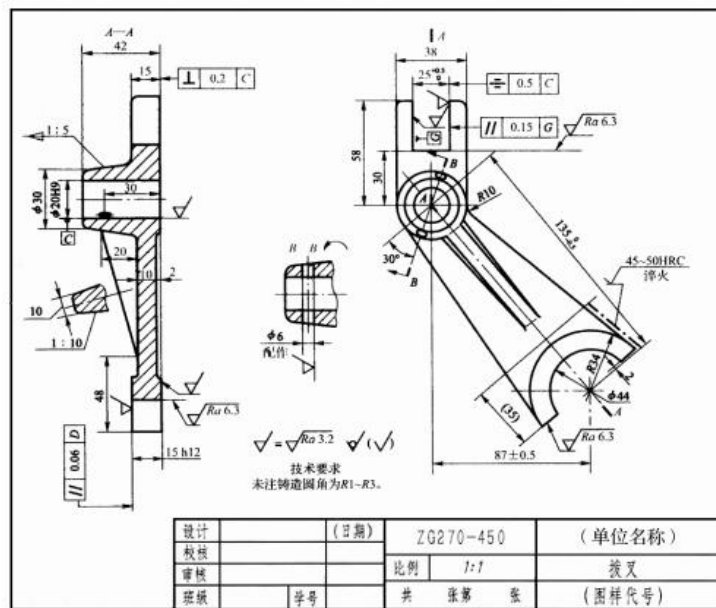
图 5-82 拨叉零件图
