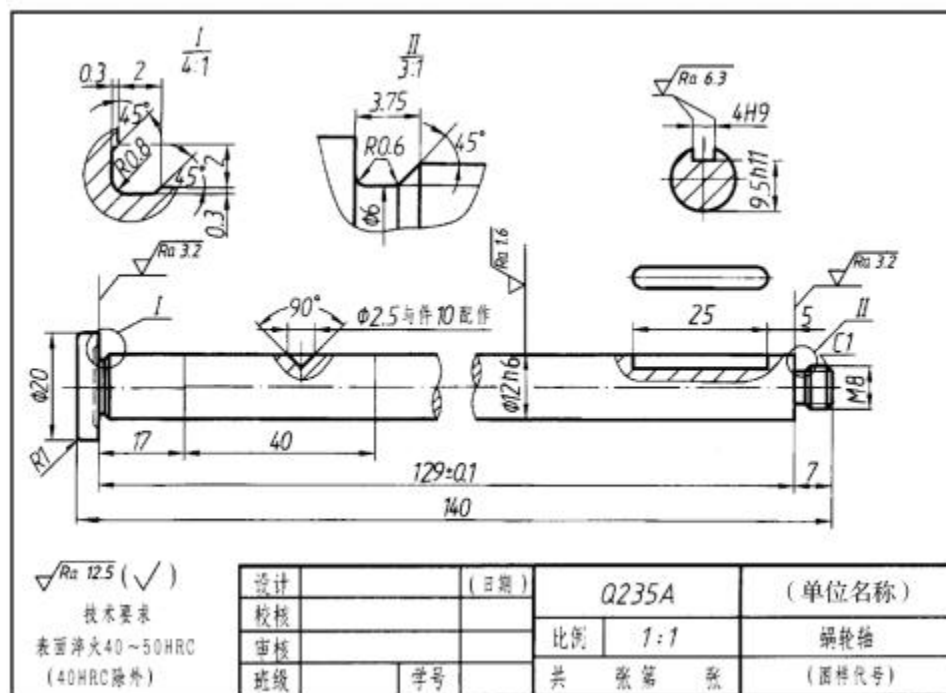
图 5-80 蜗轮轴零件图
