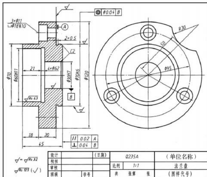
图 5-81 法兰盘零件图
