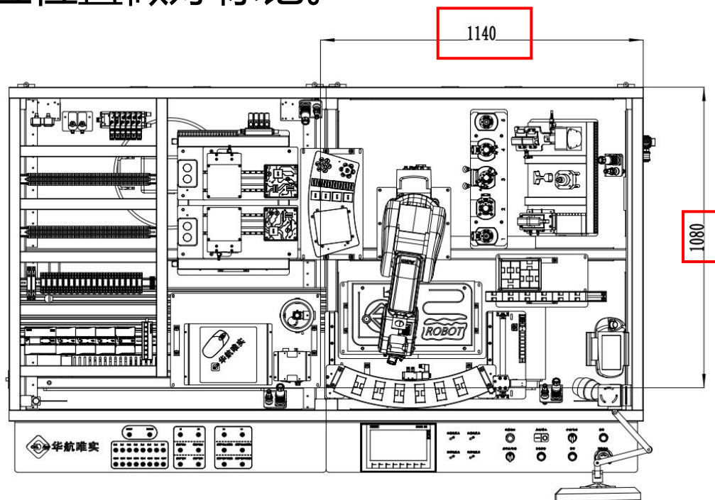
工作站机械布局图
