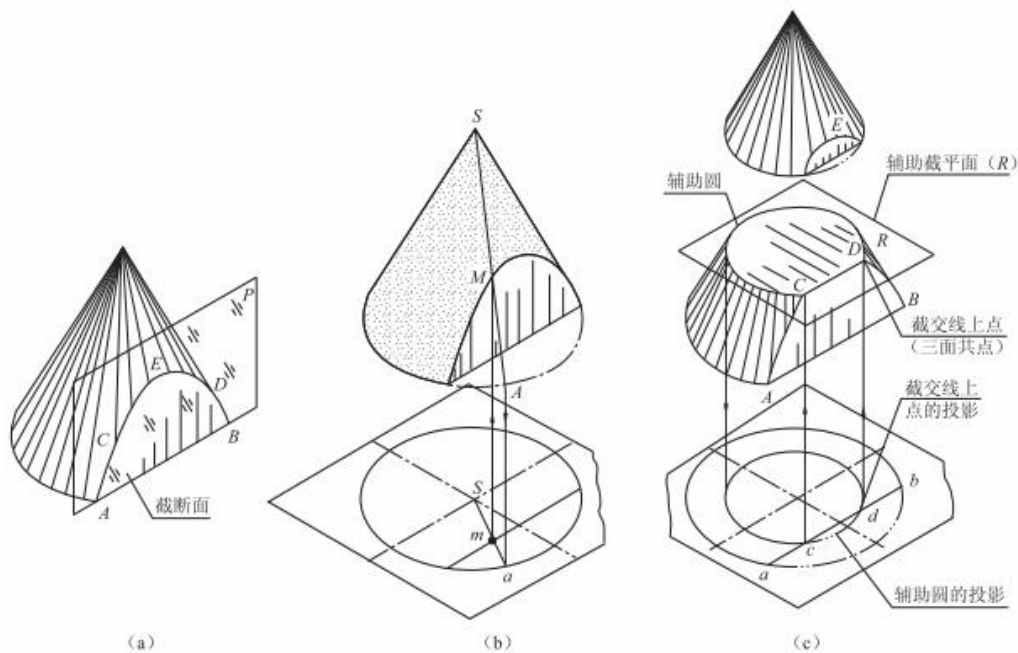
图 3-5 求圆锥表面截交线方法
