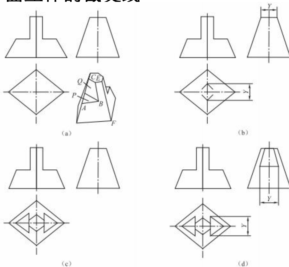
图 3-2 棱锥的切割体画图步骤
