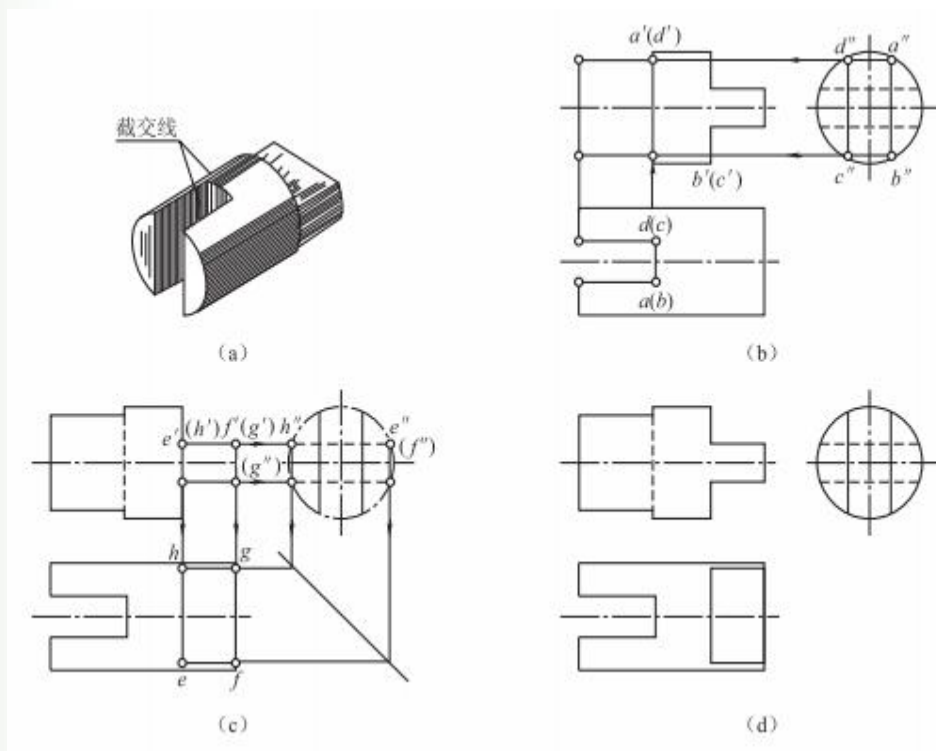
图 3-4 圆柱截交线的作图步骤
