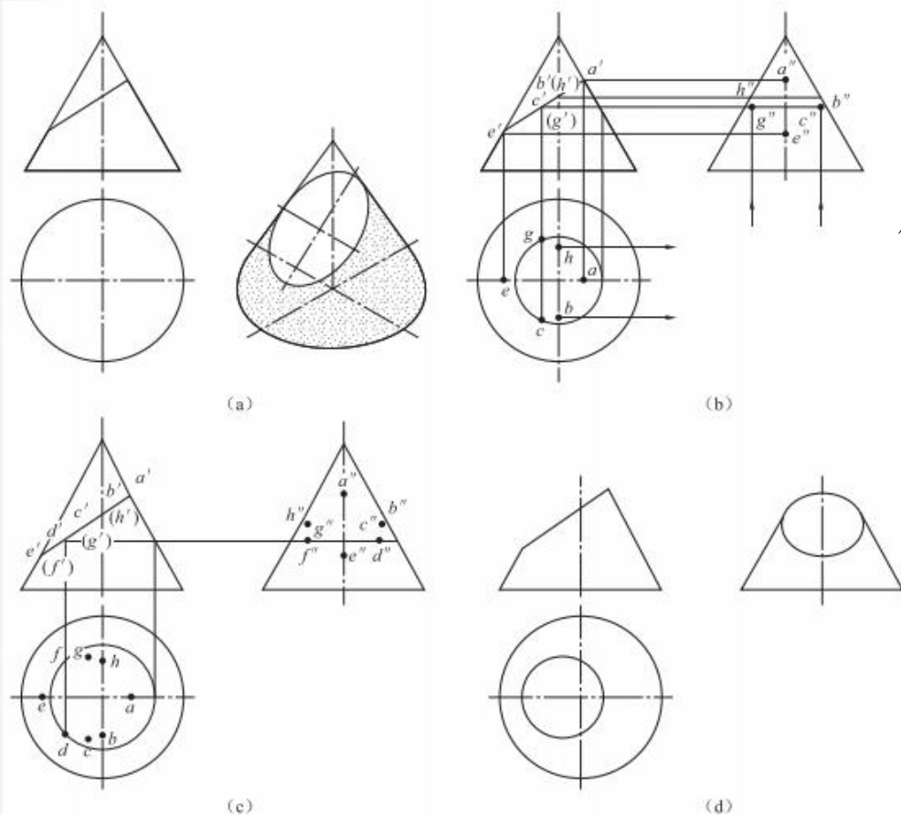
图 3-6 求圆锥表面截交线方法
