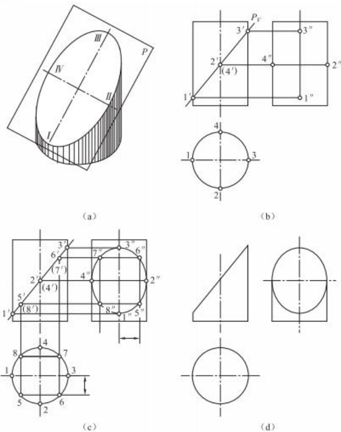
图 3-3 圆柱截交线的作图步骤
