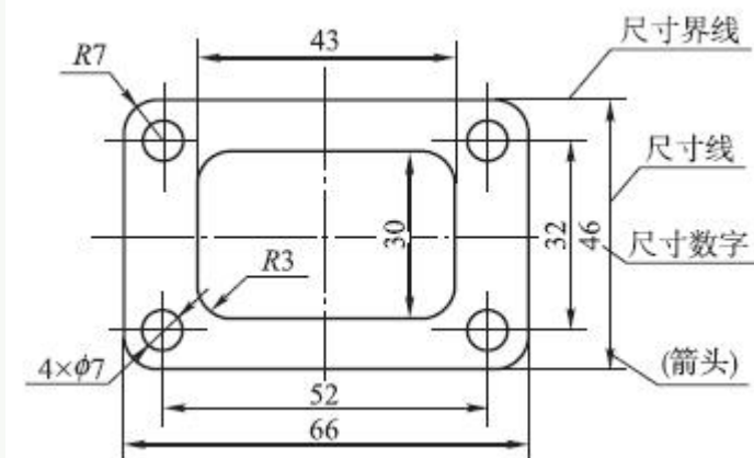
图 1-20 标注尺寸的要素
