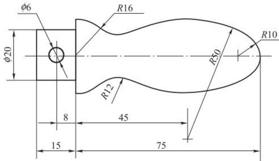
图 1-22 平面图形的尺寸分析与线段分析
