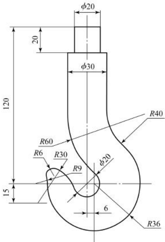
图 1-9 吊钩
