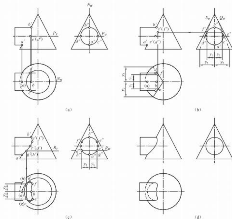
图 3-17 求圆柱与圆锥相贯线的作图过程
