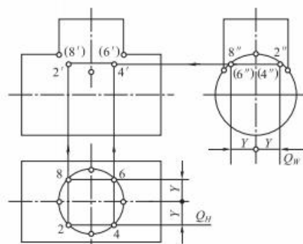
(2) 求一般点的投影
