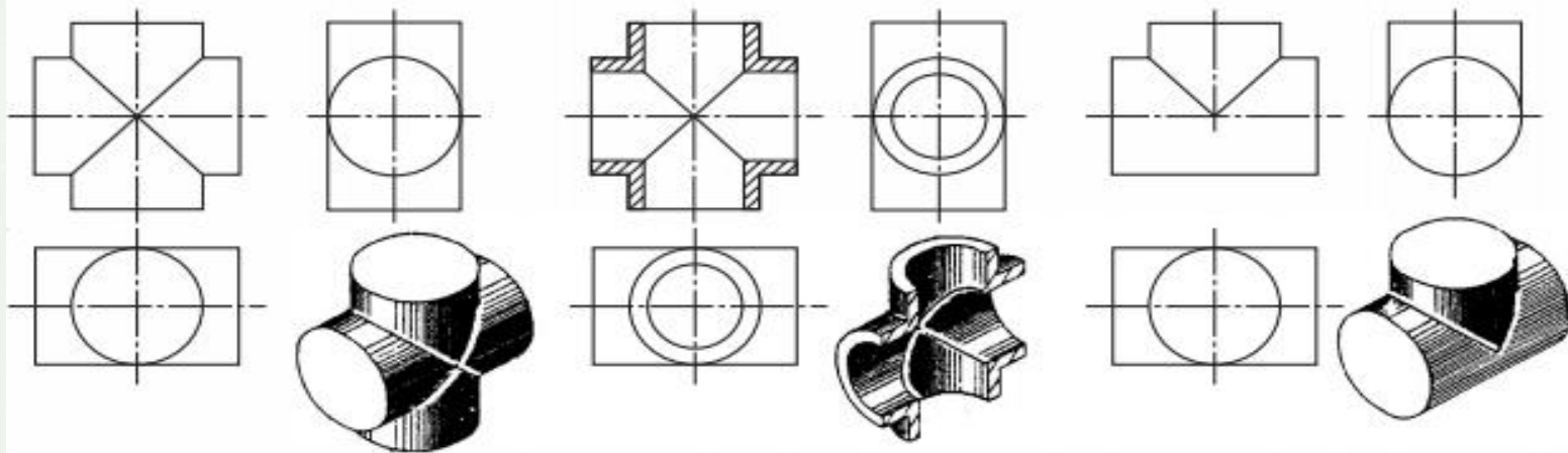
图 3-14 直径相等圆柱的相贯线
