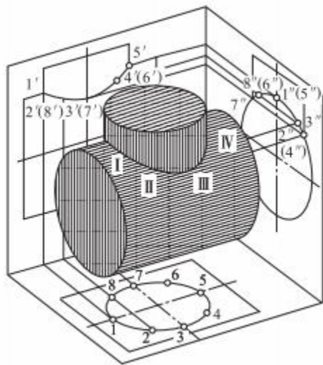
图 3-12 两圆柱相贯
