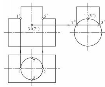
(1) 求特殊点的正面投影
